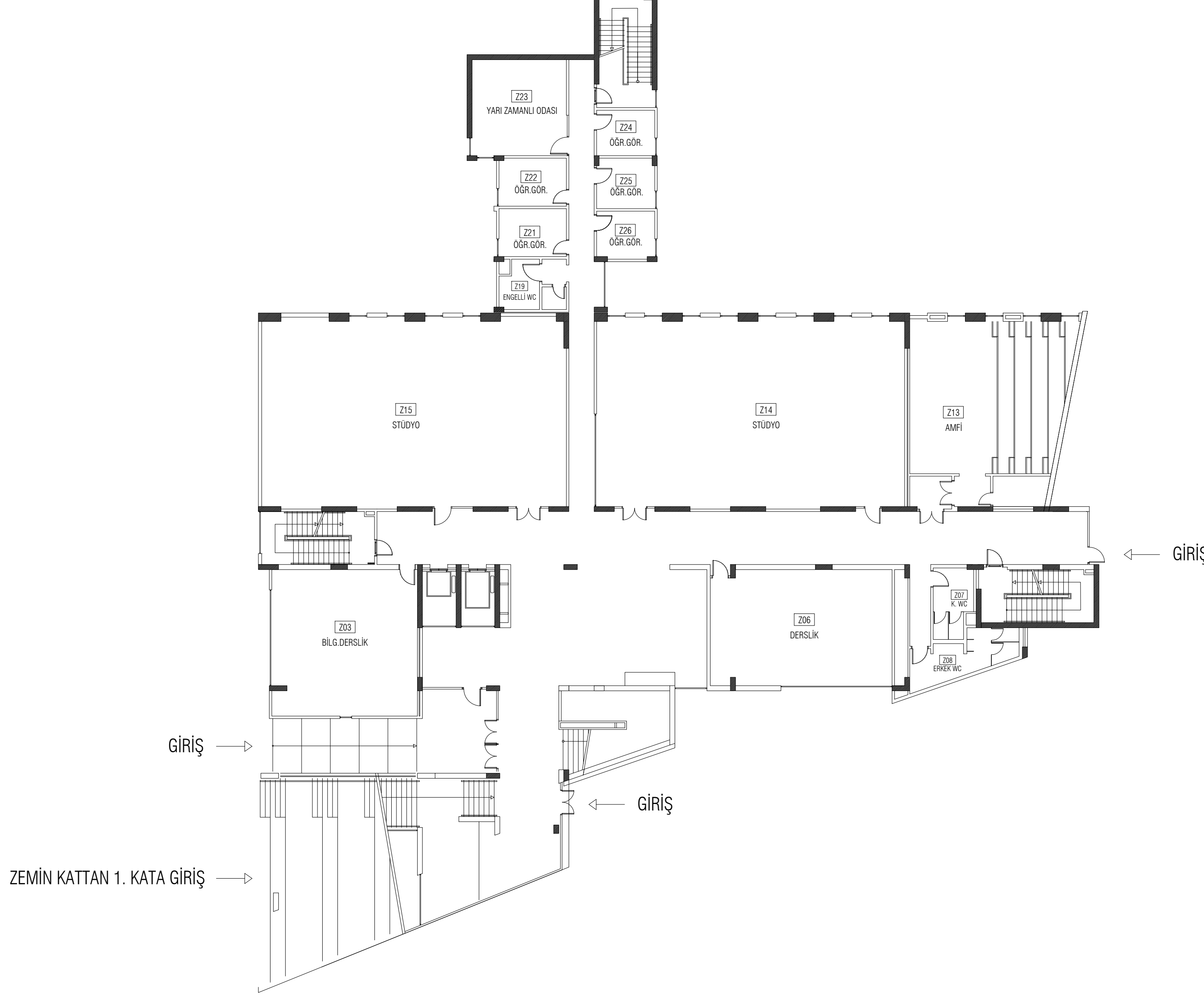
ZEMİN KAT PLANI
